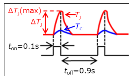
\Delta T_j パワーサイクル試験波形
