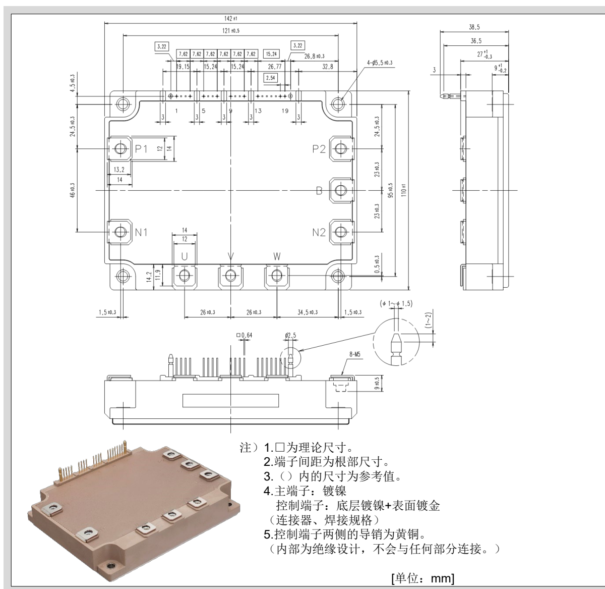
图1-9外形图（P631）
