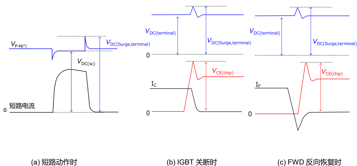
图. 1-5 集电极-发射极电压
