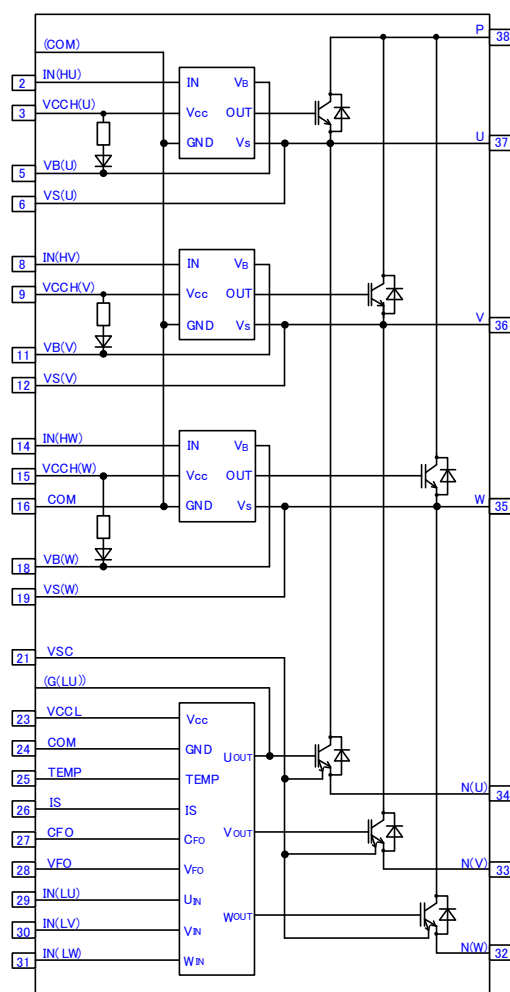
图.1-1 内部电路图
