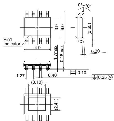
SOP-8E
