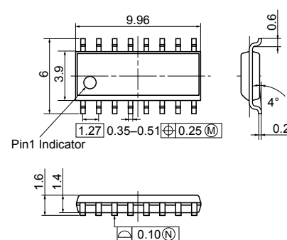
SOP-16(N)
