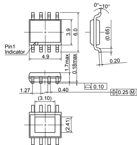
SOP-8E
