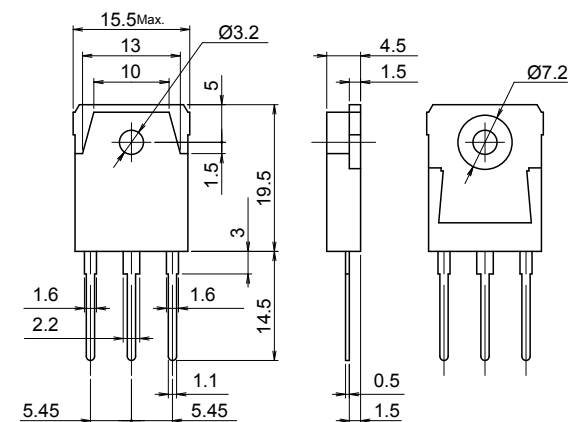
TO-3P(Q)
