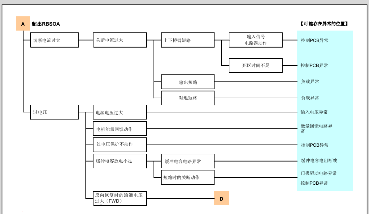
(a) 模式A: 超出RBSOA
