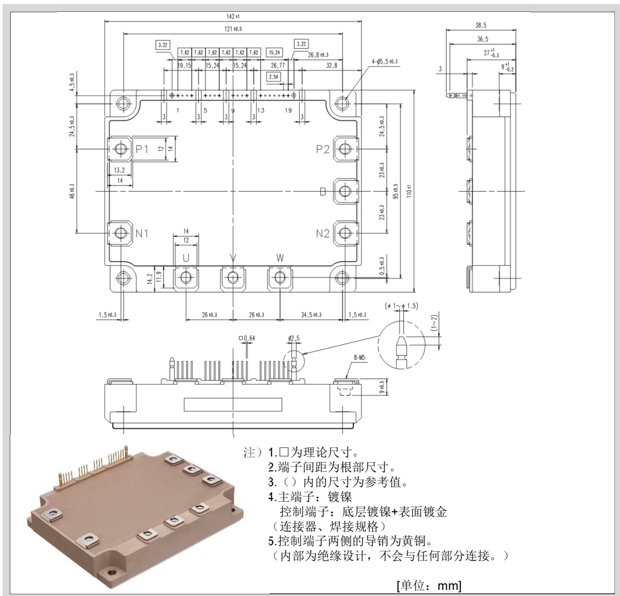
图1-9外形图（P631）
