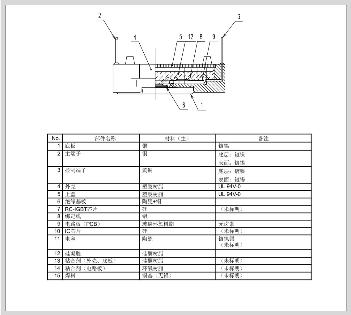
图1-10 构造（P639）
