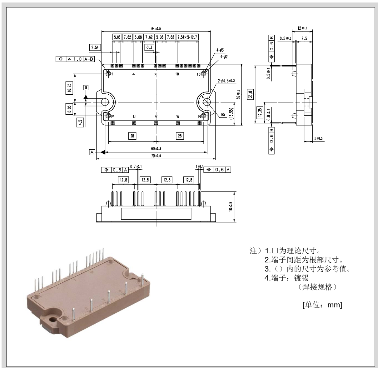
图1-2外形图（P639）
