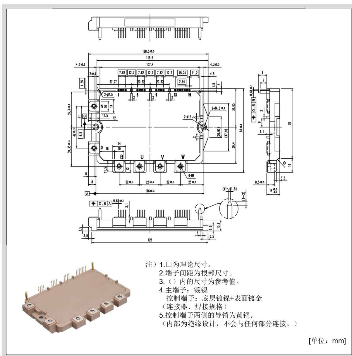
图1-8外形图（P630）
