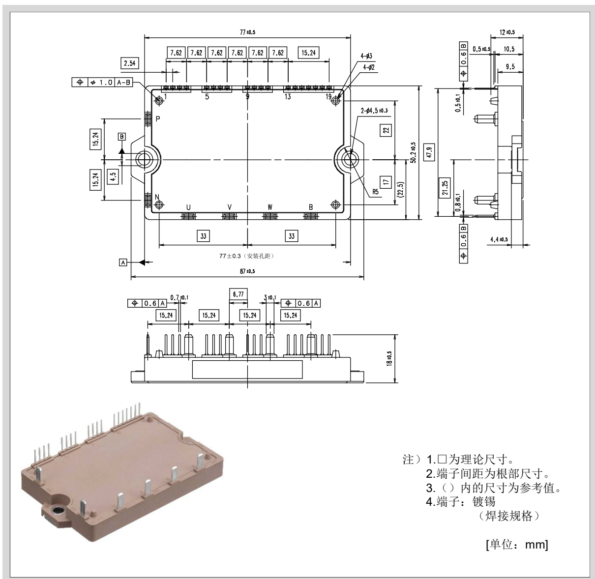
图1-5外形图（P644）
