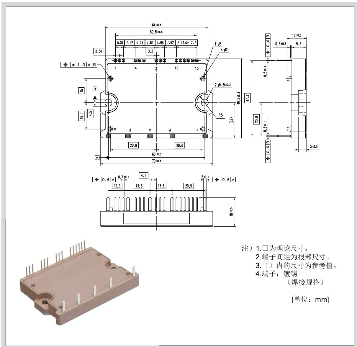
图1-3外形图（P629）
