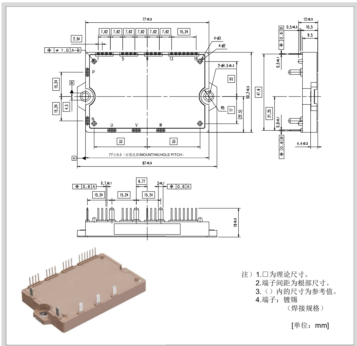
图1-4外形图（P626）
