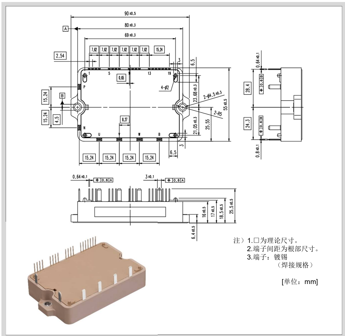
图1-6外形图（P636）
