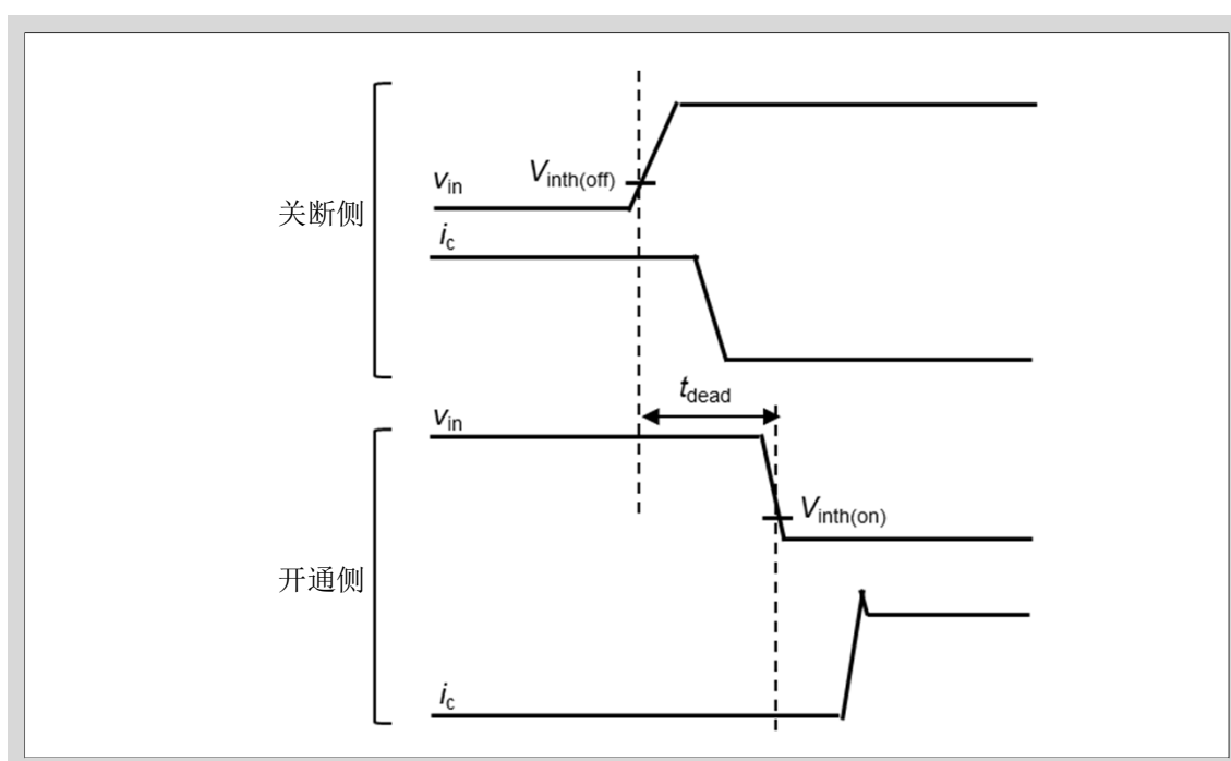
图2-6 死区时间
