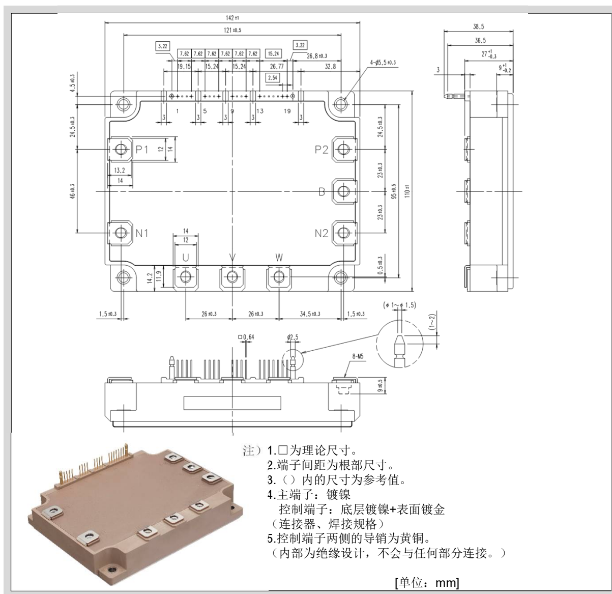
图1-9外形图（P631）
