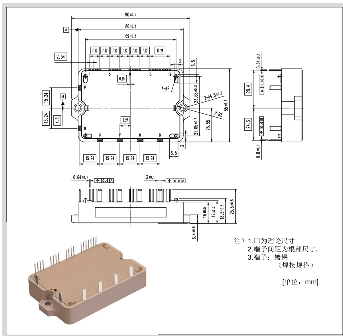
图1-6外形图（P636）
