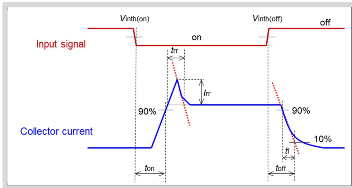
图2-1 开关时间
