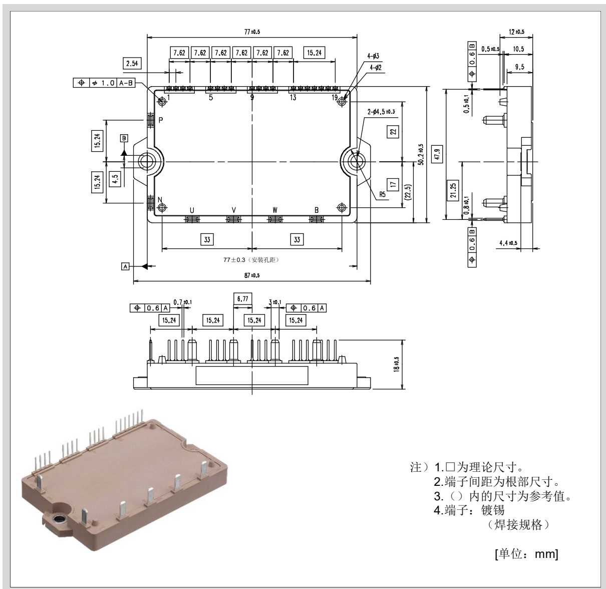
图1-5外形图（P644）
