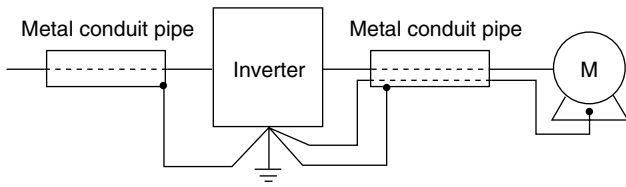
Fig. 8 Grounding of metal conduit pipe
